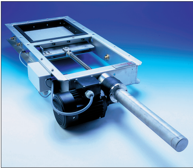
Elektrisk drift.
